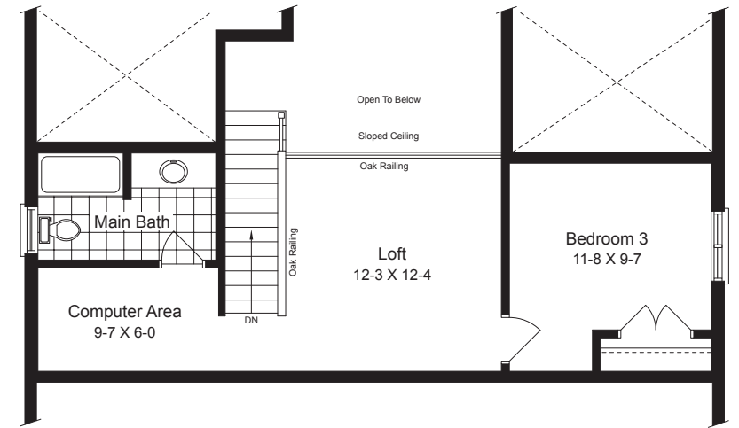
OPTIONAL LOFT FLOORPLAN
